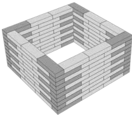
„Basilikum“ 120x120x60 cm Pflanzfläche ca. 0,92 m 2
